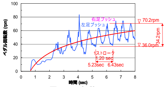
図-5.1 回転数
