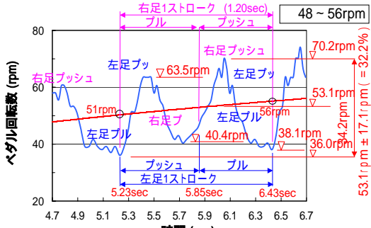
図-5.2 回転数
