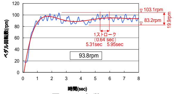
図-6.1 回転数
