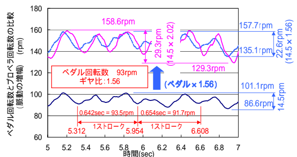
図-7 回転数の比較
