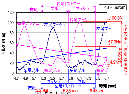
図-5.3 トルク
