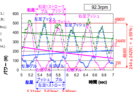
図-6.4 パワー
