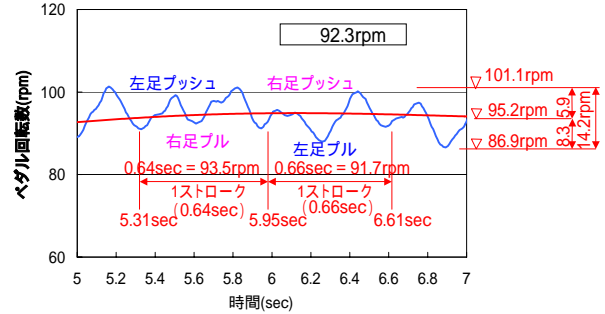
図-6.2 回転数
