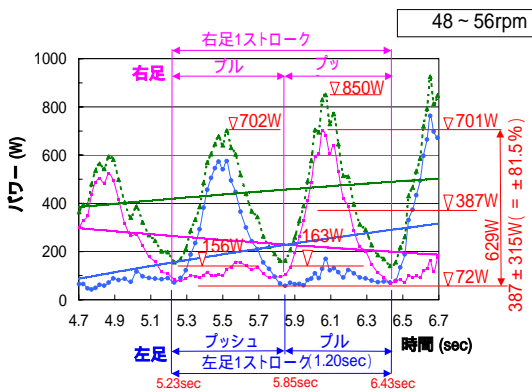
図-5.4 パワー
