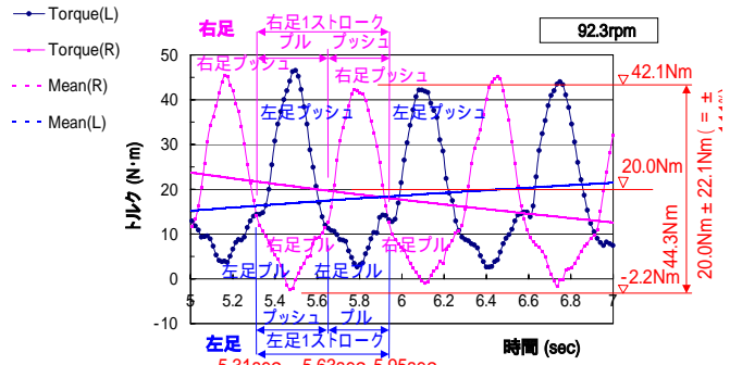
図-6.3 トルク
