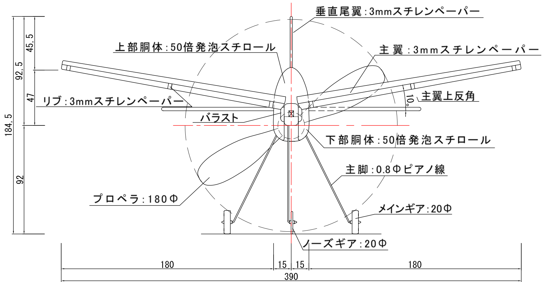
正面図 縮尺: 1/2
