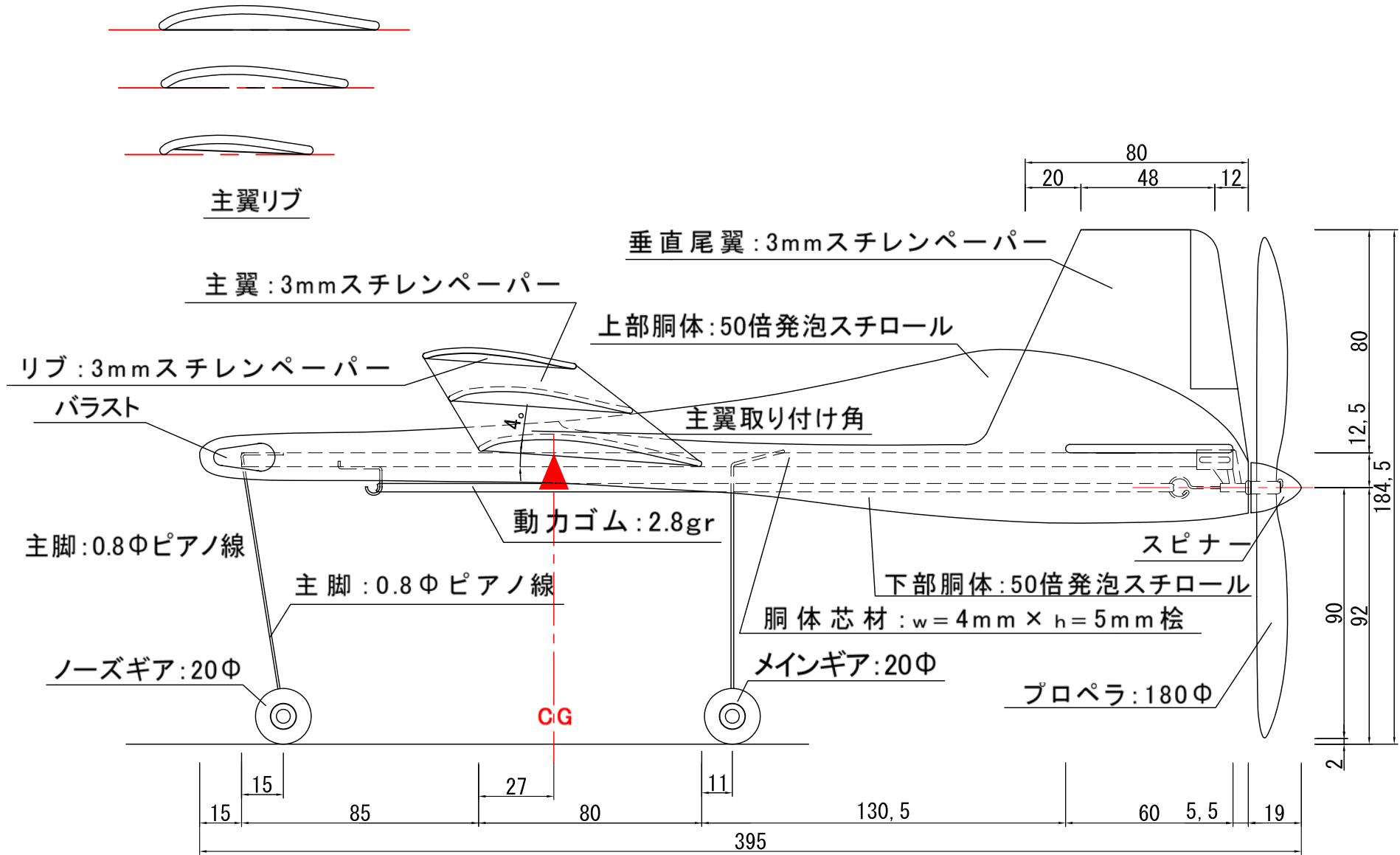
側面図 縮尺: 1/2
